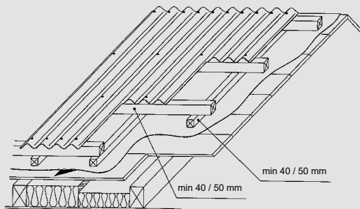
Slika 1.: Primer izoliranega ostrešja
