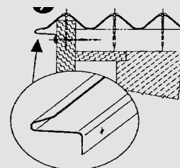
Slika 3.: Primer zaključka s pocinkanimi vetrnimi obrobami iz našega programa. Glejte stran 5.
