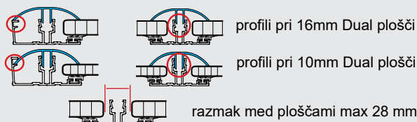
ALU-PVC profili v prerezu
